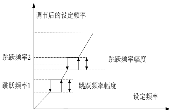
图 6-8 频率跳跃示意图
