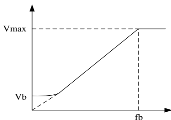
图 6-3 转矩提升示意图
