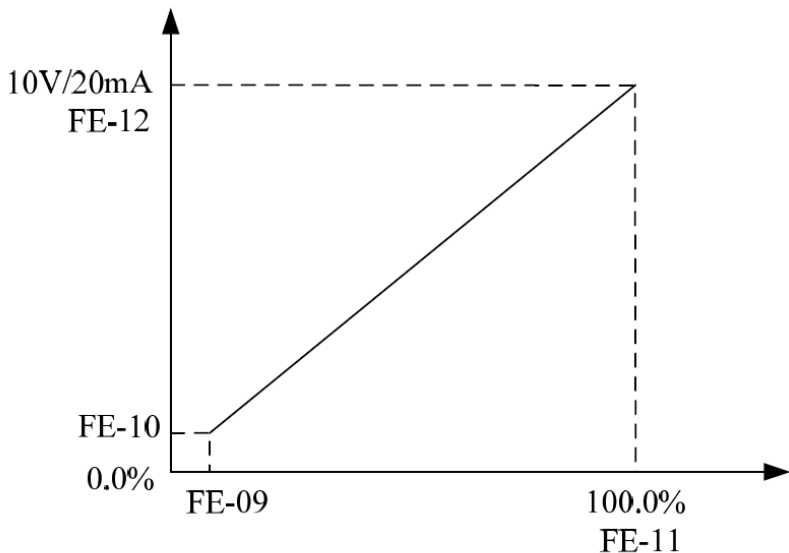
图 6-30 模拟 AOV/AOI 线性比例图
