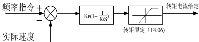
图 6-11 速度环简化框图
