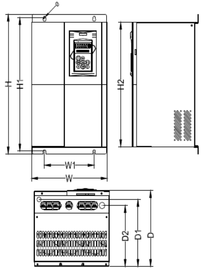
(d) 18.5-200kw 外形尺寸
