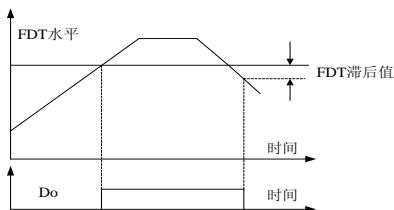
图 6-19 频率水平检测示意图
