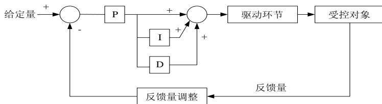
图 6-23 PID 系统结构图
