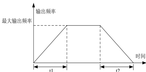
图 6-2 加速时间和减速时间设置说明
