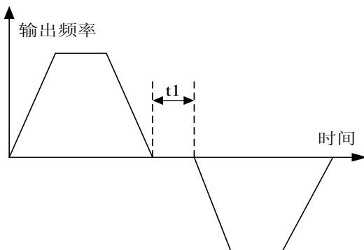
图 6-9 正反转死区时间
