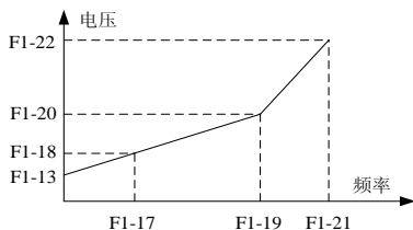
图 6-5 V/F 自定义曲线
