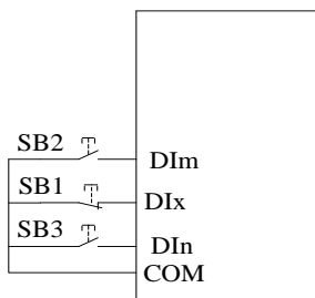
图 6-18 三线式控制 2
