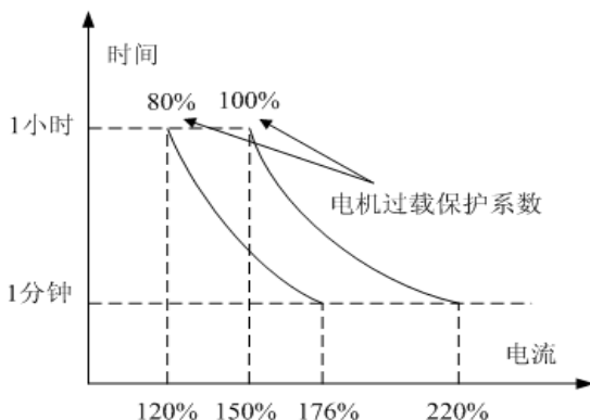
图 6-28 电机过载保护系数设定
