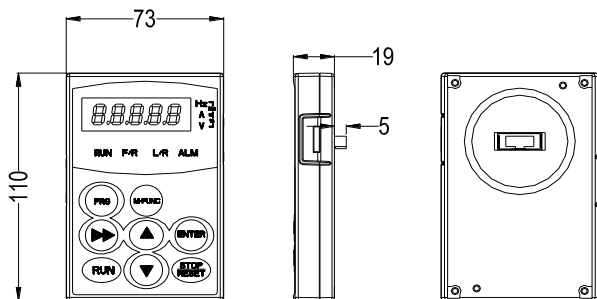
图 2-2 ETD200-LKD 键盘（本机 and 遥控）尺寸
