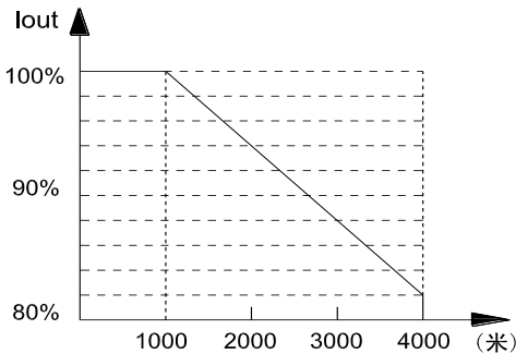
图 1-4 变频器额定输出电流与海拔高度降额使用图
