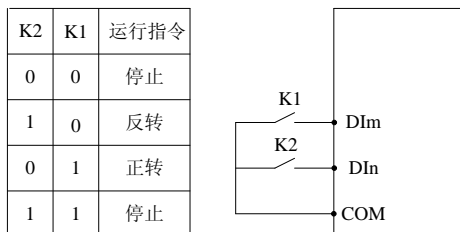
图 6-15 二线式运转模式 1
