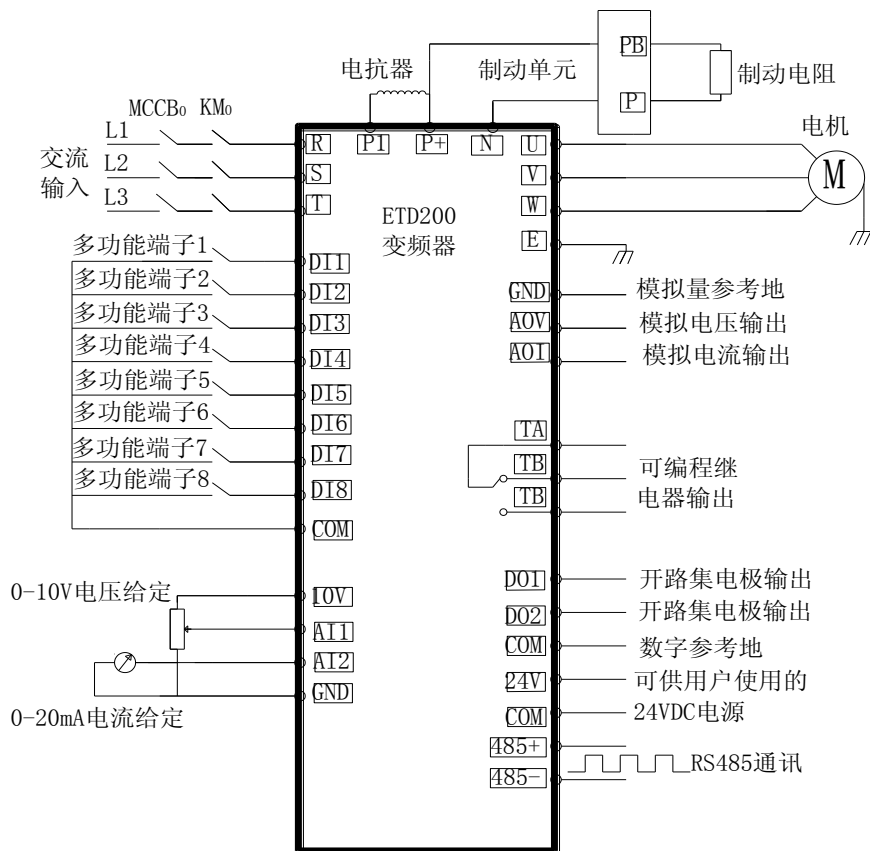
图3-14 基本运行配线图
