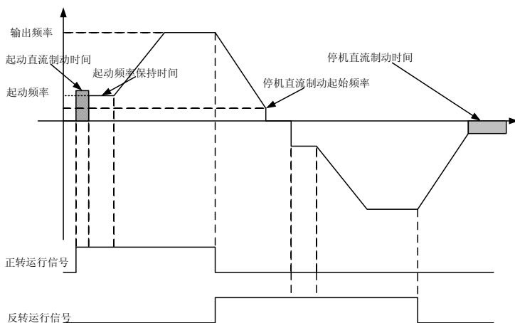
图 6-6 起动方式 1 示意图
