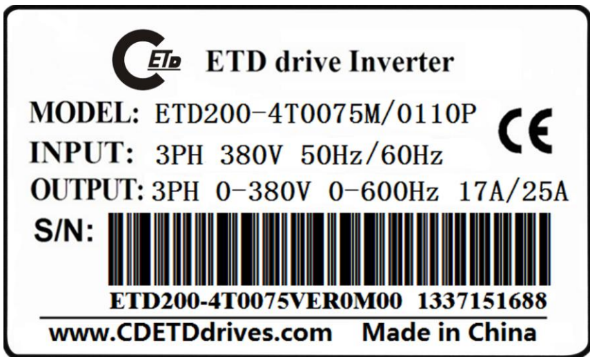
图 1-2 变频器铭牌
