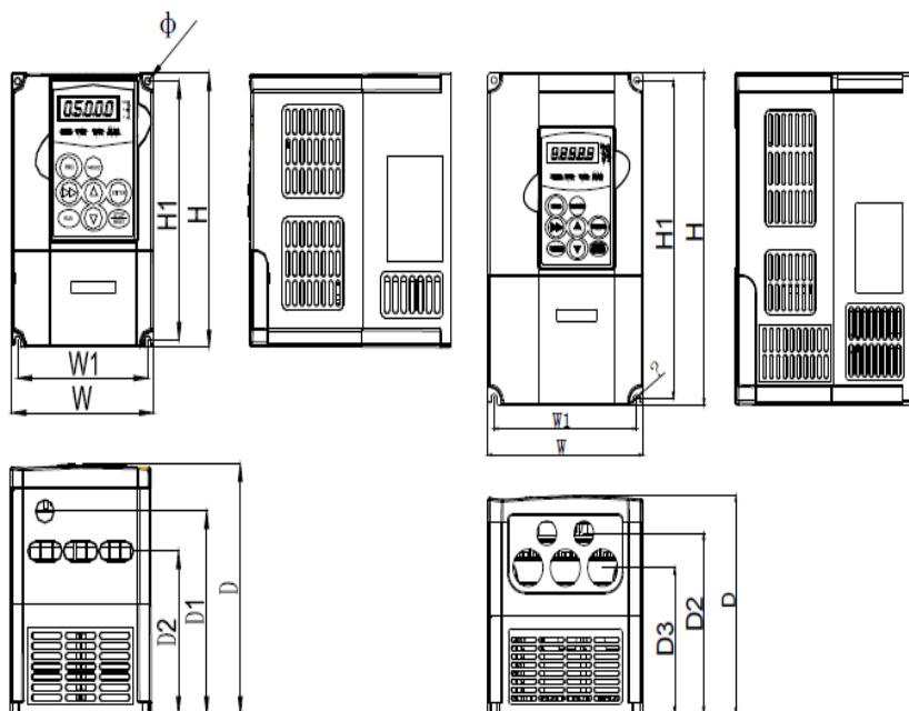
(a) 0.75-4KW 外形
