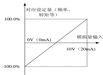
图 6-13 模拟 AI1/AI2 线性比例图
