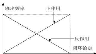
图 6-24 PID 反馈调节示意图
