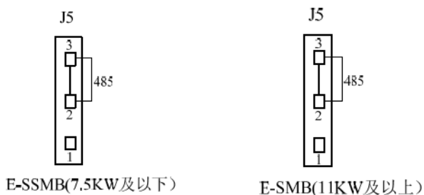
图 3-19 通讯输出端子配线图
