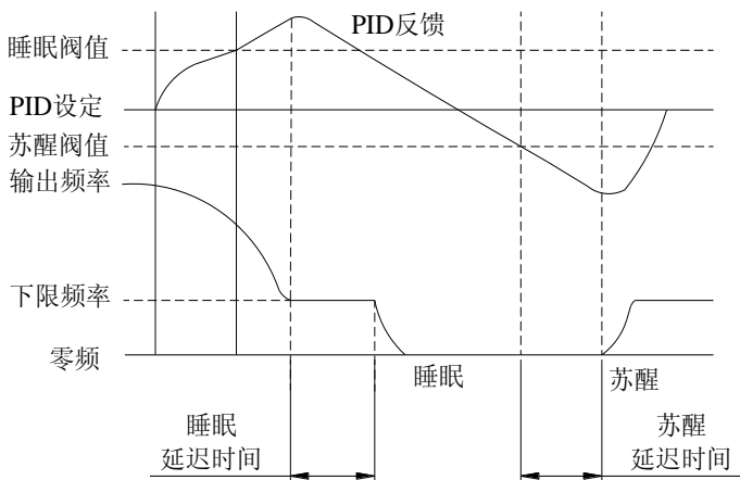
图 6-26 睡眠与苏醒功能示意图
