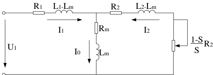
图 6-10 异步电机稳态等值电路图
