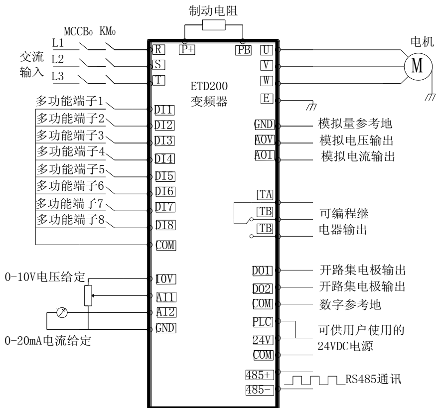
图3-13 基本运行配线图
