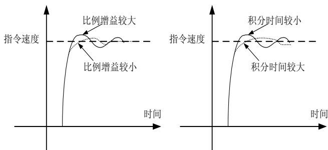
图 6-12 速度环 (ASR) 的阶响应与 PI 参数的关系
