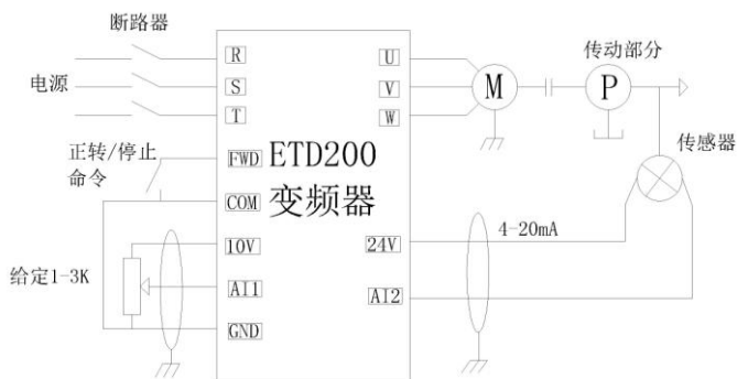
图 6-22 （FWD 端子由用户自行定义）
