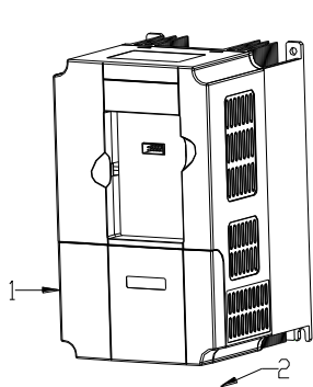
图 3-5 盖板的拆卸
