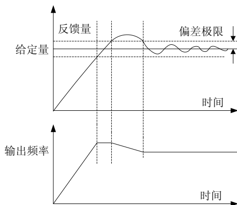
图 6-25 偏差极限示意图
