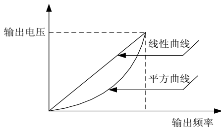
图 6-4 V/F 曲线
