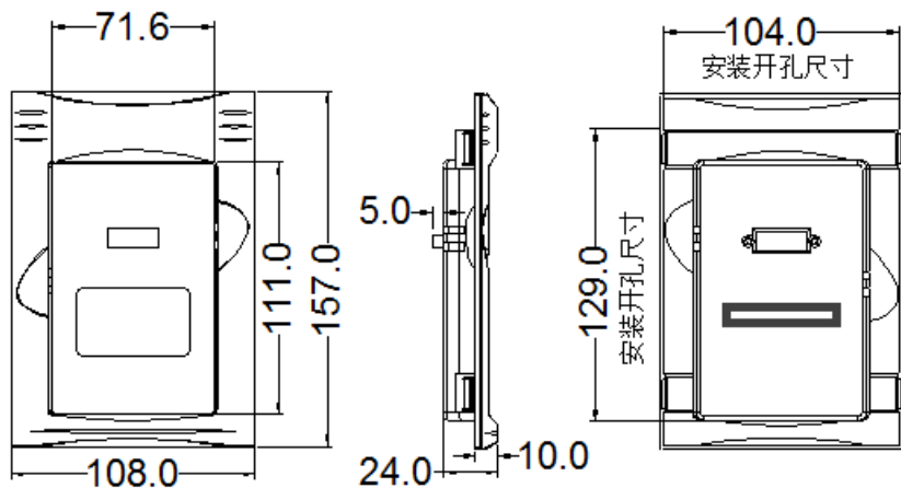
图 2-1 ETD200-LKD 遥控键盘托板尺寸（选配件）
