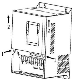
图 3-9 上盖板的拆卸
