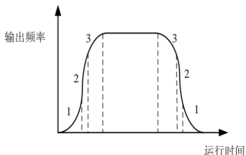
图 6-7 S 曲线加减速
