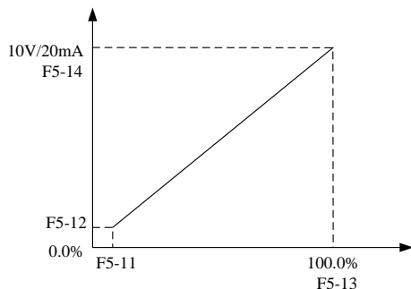
图 6-14 模拟 AOV/AOI 线性比例图
