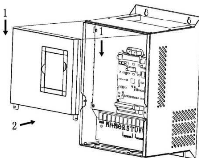
图 3-10 上盖板的安装
