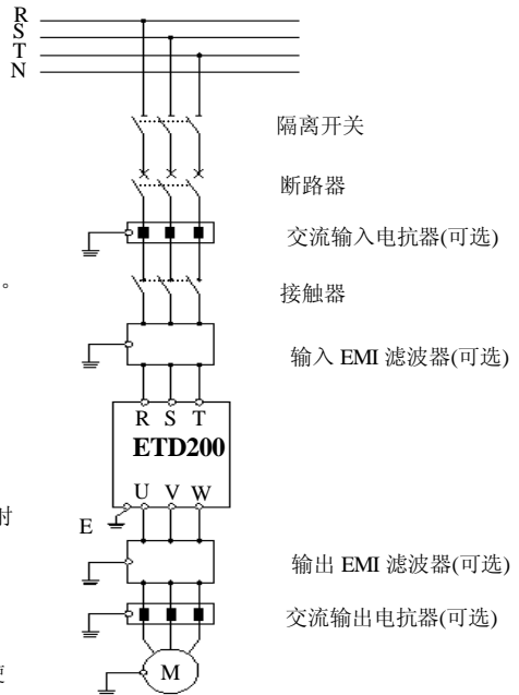
图 3-12 变频器与选配件的连接
