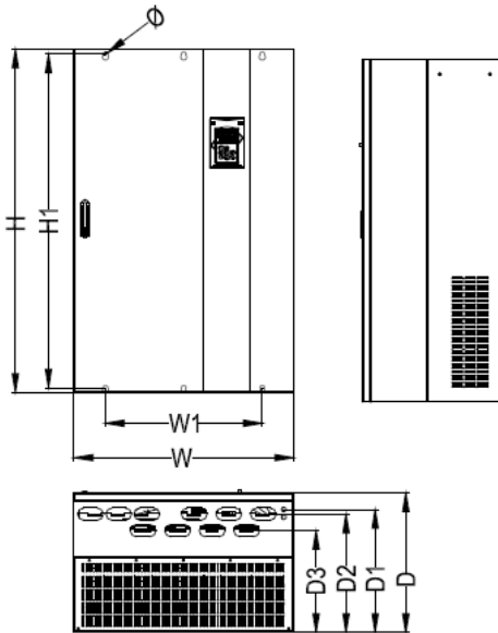
(c) 11-15KW 外形尺寸
