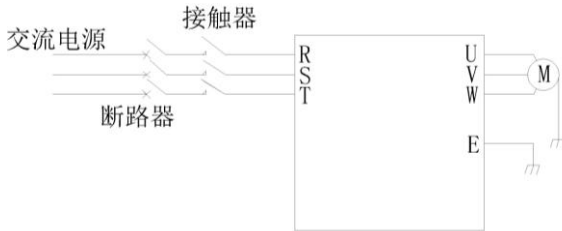
图 3-11 主回路简单配线
