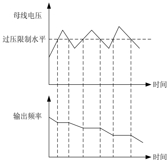
图 6-29 过压限制水平说明
