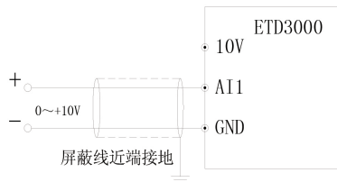
图 3-21 AI1 端子配线图
