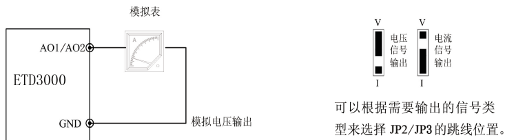
图 3-23 模拟输出端子配线
