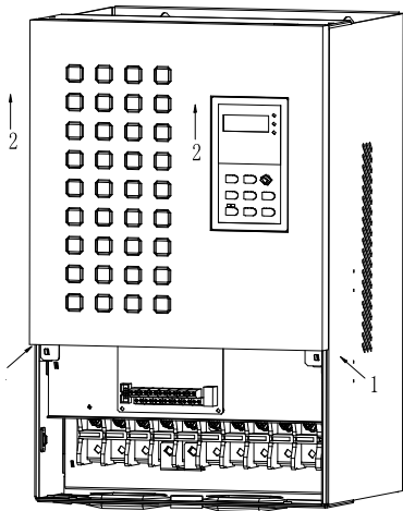
图 3-9 盖板的拆卸
