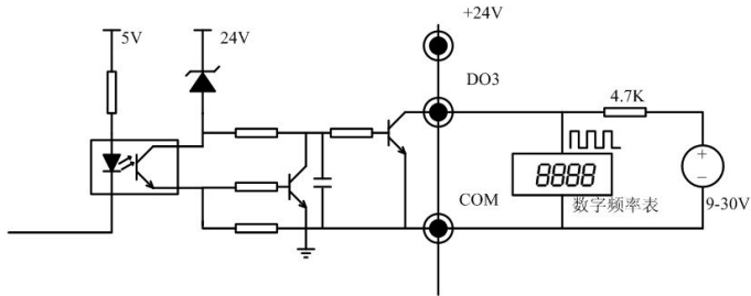
DO3 端口使用变频器外部电源的外部接线示意图
