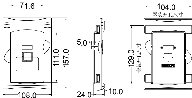
图 2-3 ETD3000-RKB 托板尺寸 (RKB键盘选配件)
