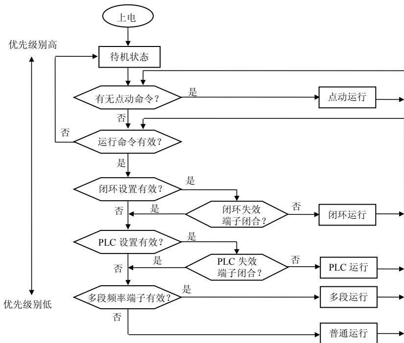
图 4-1 ETD3000变频器运行状态的逻辑关系图
