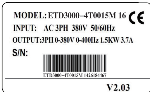
图 1-2 变频器铭牌
