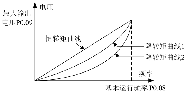
图 6-4 V/F 曲线
