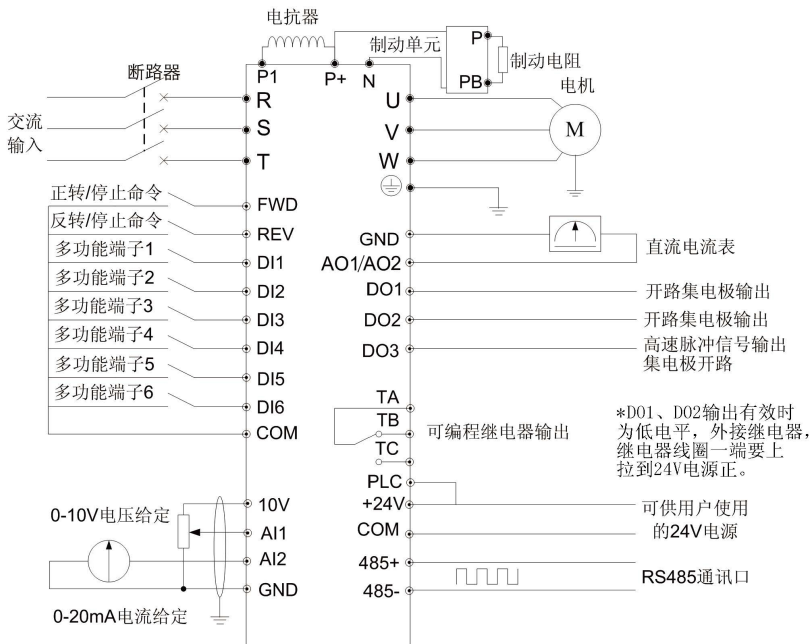
图 3-18 基本运行配线图
