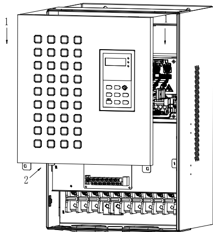
图 3-10 盖板的安装
