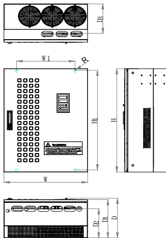
(d): 93KW~200KW 规格尺寸(壁挂)
