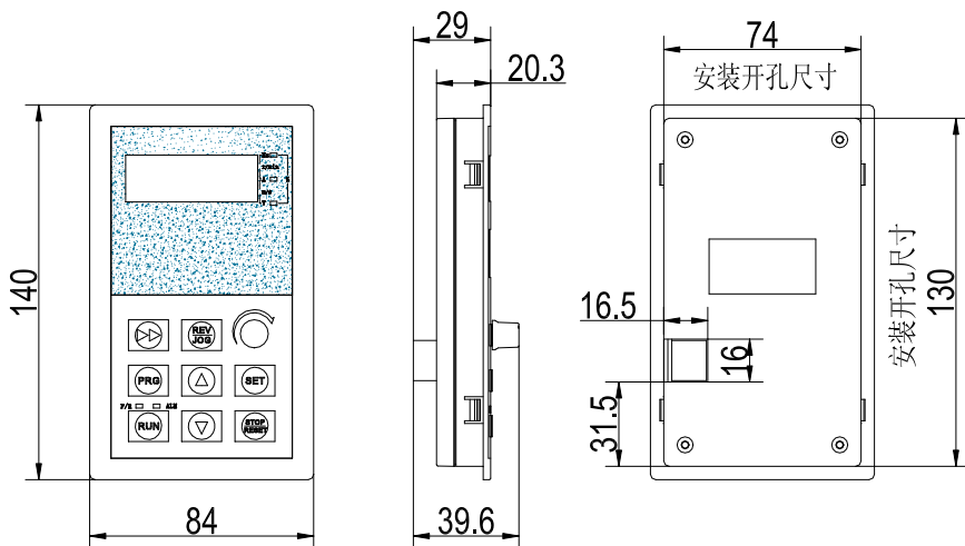
图 2-1 ETD3000-LKD 外引托板尺寸 (选配件)
