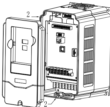
图 3-6 盖板的安装
