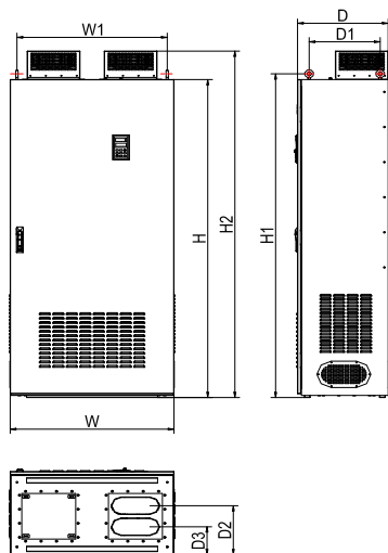
(h): 315KW~400KW 规格尺寸(柜机)
