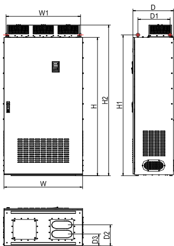
(i): 500KW~630KW 规格尺寸(柜机)
