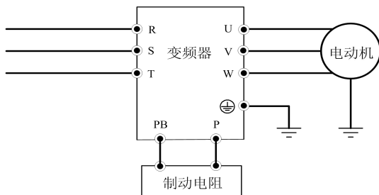
图 2-3 变频器与制动组件连线图（380V 18.5KW 以下）
