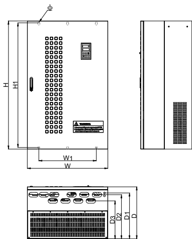
(e): 220KW~315KW 规格尺寸(壁挂)
