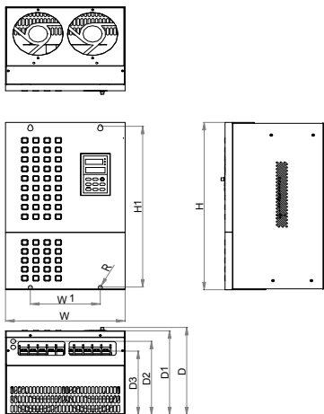
(c): 11KW~75KW 规格尺寸
