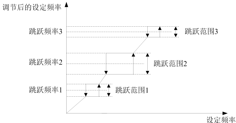
图 6-10 跳跃频率设定
