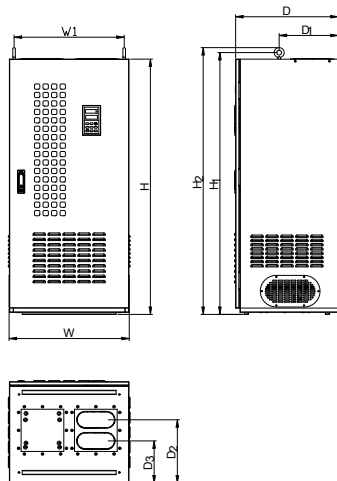
(f): 160KW~200KW 规格尺寸(柜机)
