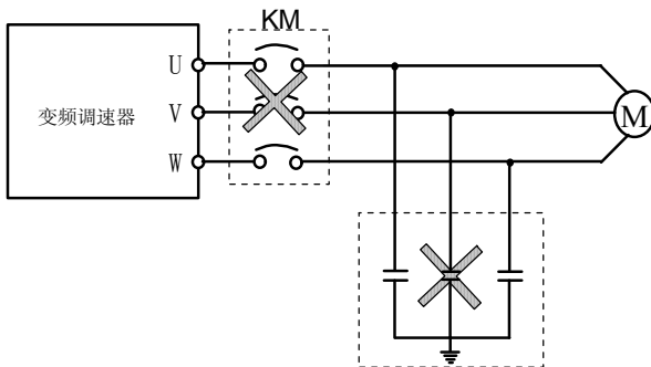
图 1-3 变频器输出端禁止使用电容器
