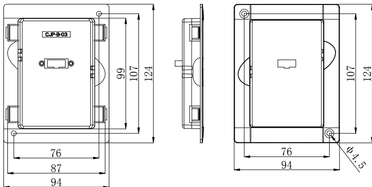
图 2-1 ETD3000-LKD 外引托板尺寸 (选配件)
