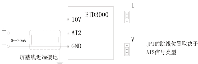
图 3-22 AI2 端子配线图
