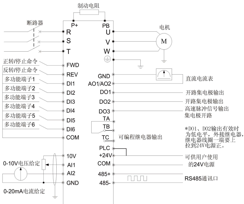
图 3-17 基本运行配线图
